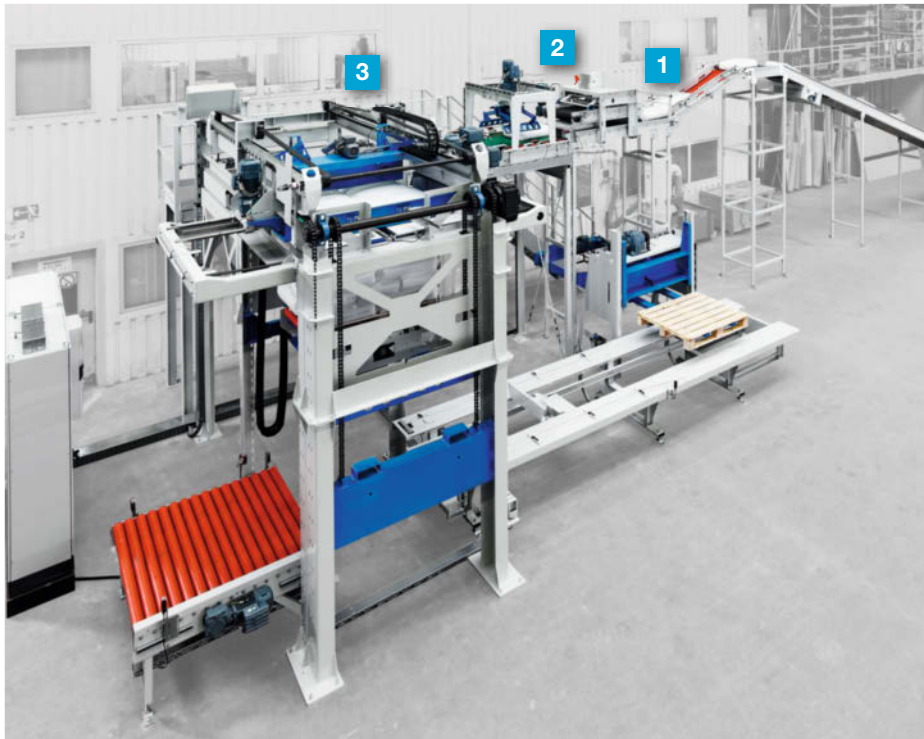
BEUMER Doppelband-Drehvorrichtung
